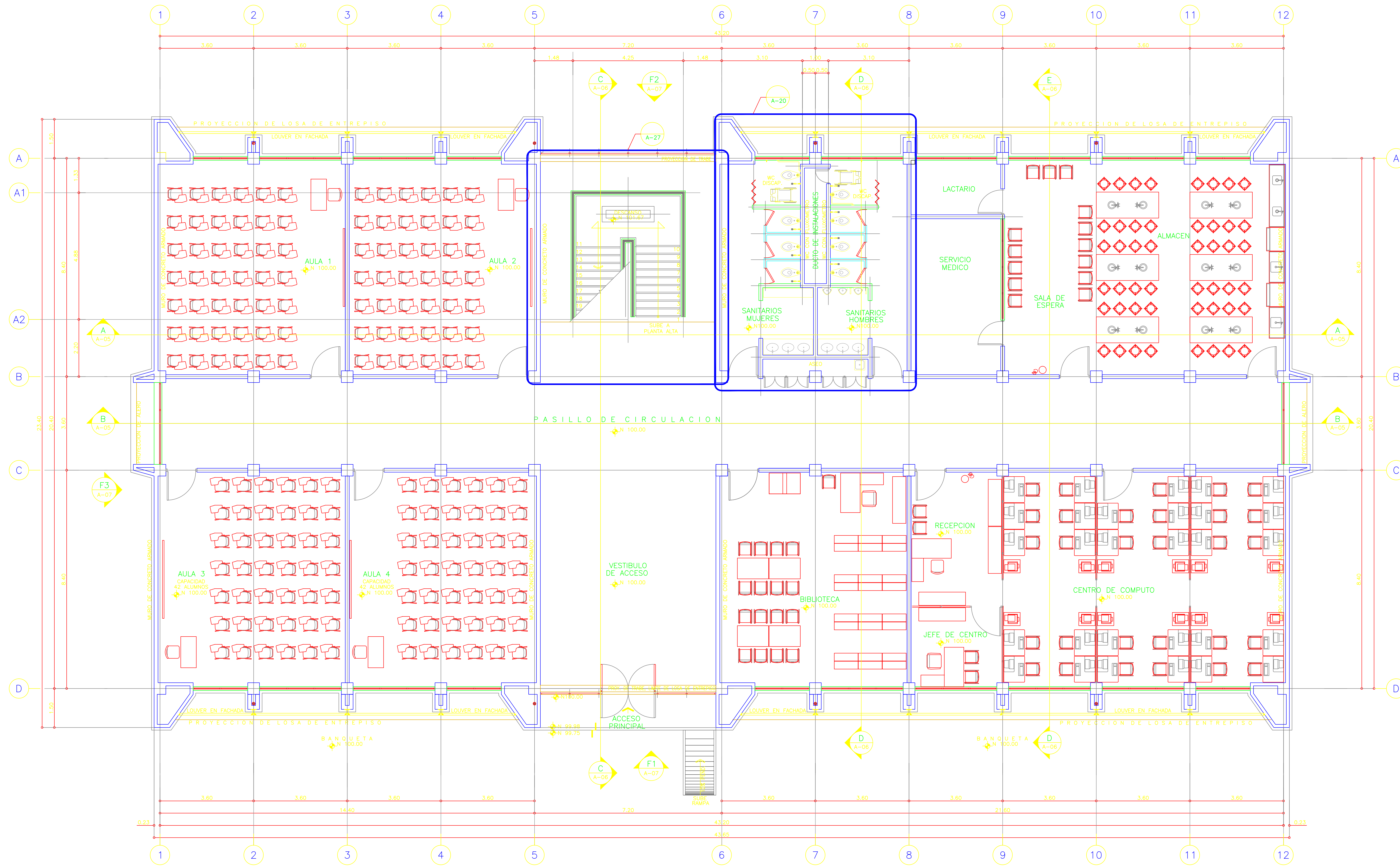
ARQUITECTONICO -PLANTA BAJA ESCALA 1:75 COTAS EN MTS
